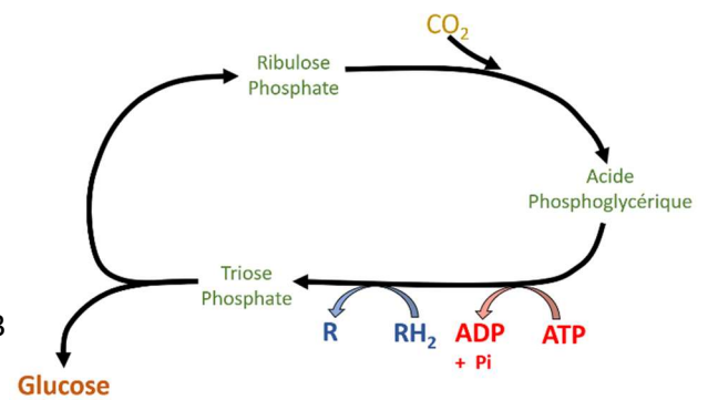
Schéma bilan de la phase non-photochimique
