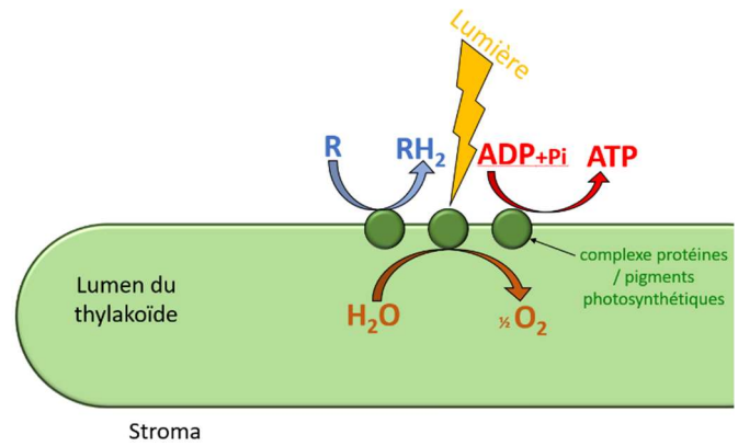
Schéma bilan de la phase photochimique
